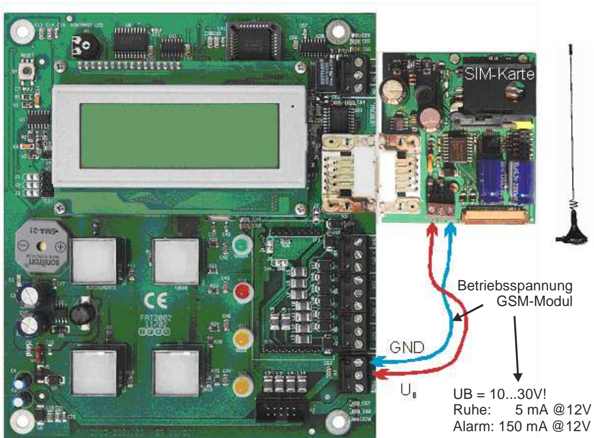
Abbildung 1 : GSM-Modul am FAT2002 (nicht redundant)
