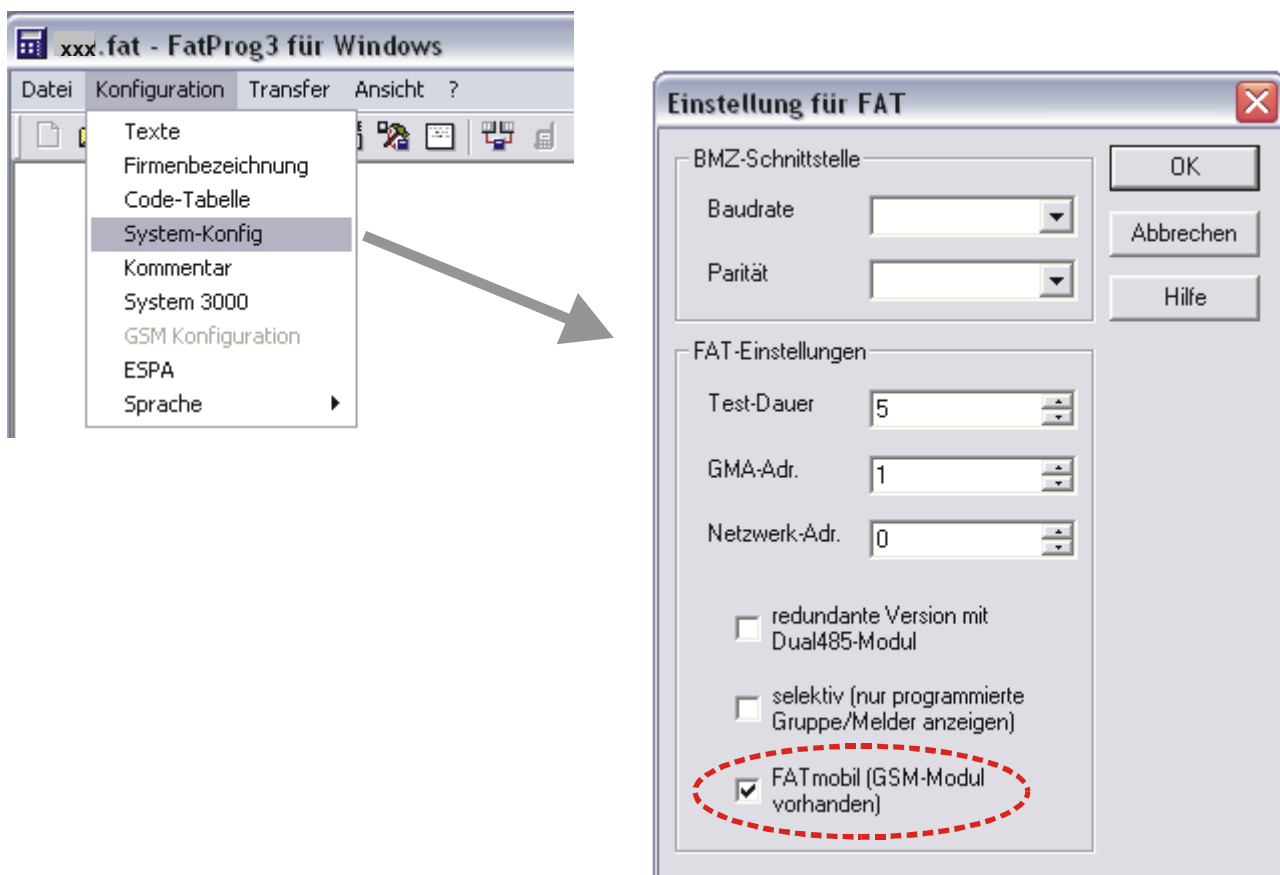
Abbildung 4 : Systemkonfiguration
