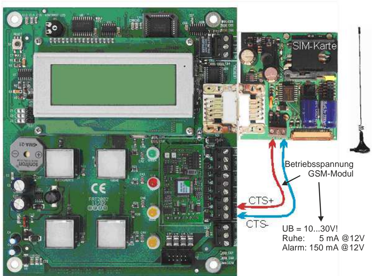
Abbildung 2 : GSM-Modul am FAT2002 RE (redundant)
